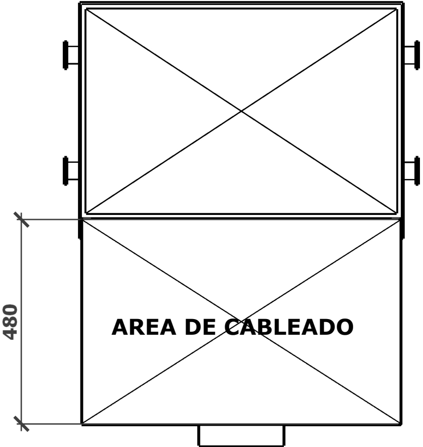
VISTA SUPERIOR
