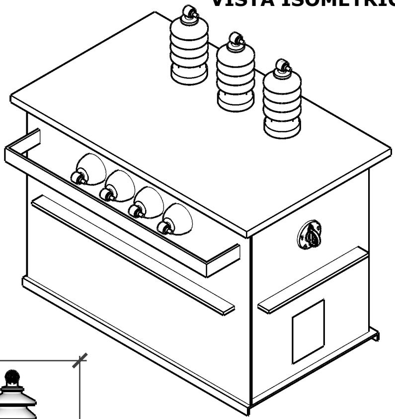
VISTA ISOMETRICA
