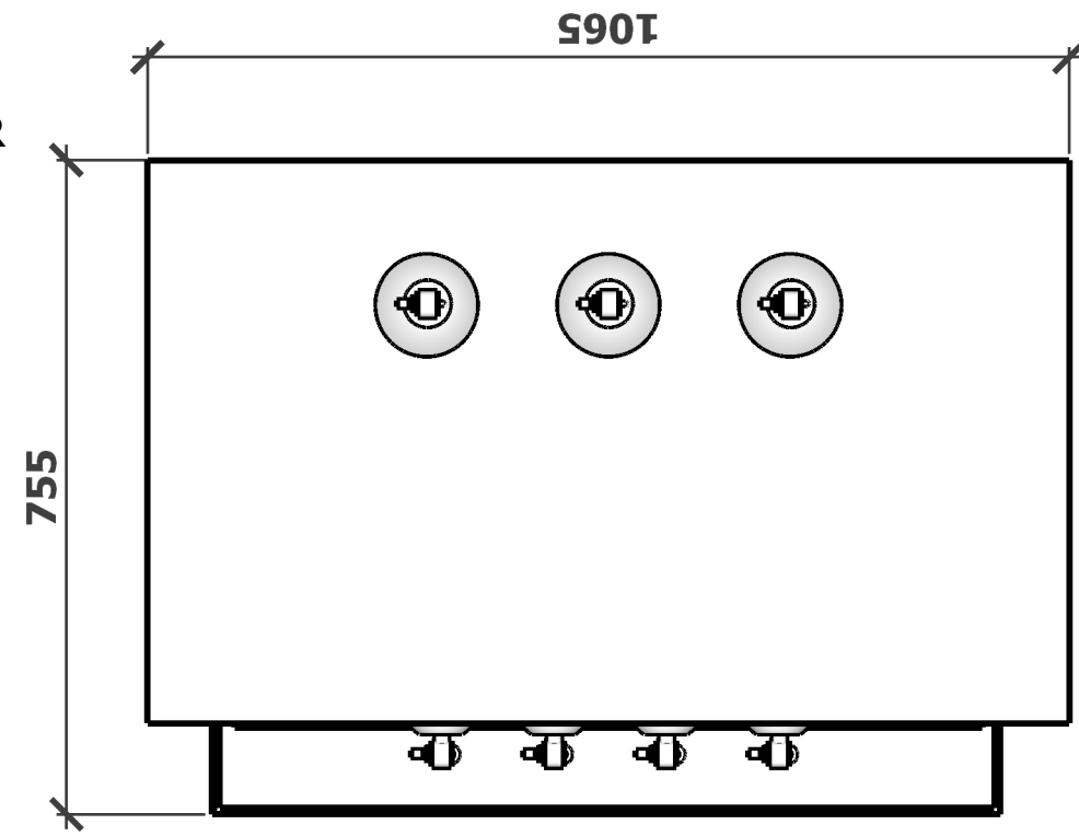
VISTA SUPERIOR
