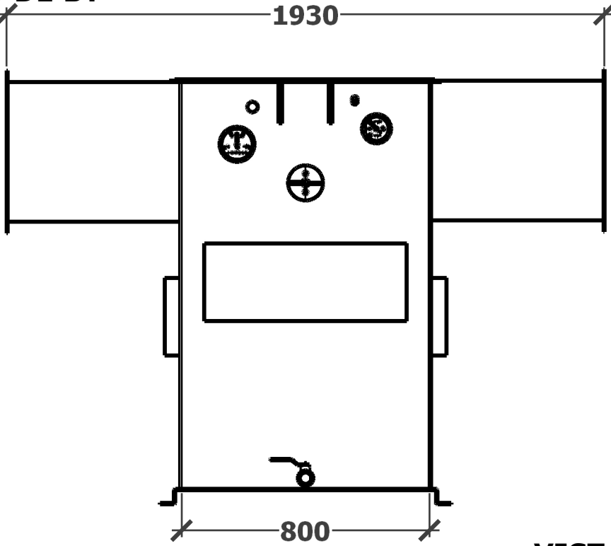
VISTA LATERAL
